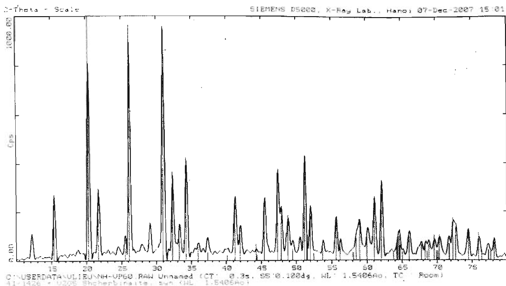
Hình 3: Giảm đồ X-ray của mẫu nung ở điều kiện tối ưu
