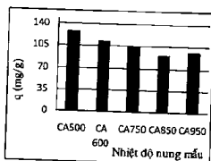
Hình 3: Sự phụ thuộc của nhiệt độ nung vật liệu \text{CeO}_2\text{-Al}_2\text{O}_3 đến dung lượng hấp phụ \text{PO}_3^-
